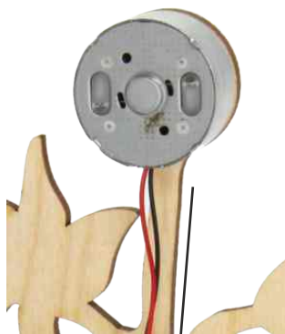
(FR) Orientation du câble du moteur (NL) Uitlijning motorkabel
